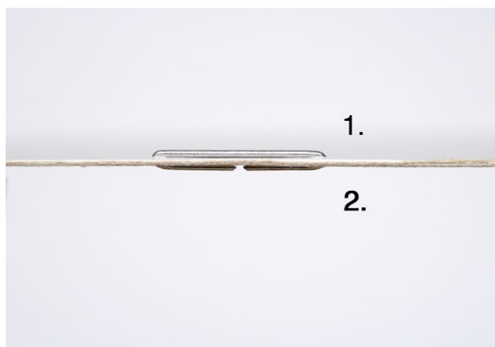
Avec les 2 nouvelles étapes d'agrafage, les pattes d'agrafe percent d'abord le papier. Les extrémités des agrafes sont ensuite repliées et pressées à plat contre le papier.
